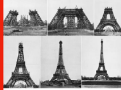
Gustave Eiffel, étapes de la construction La Tour métallique éponyme, pour l'Exposition Universelle de 1889, à Paris.
