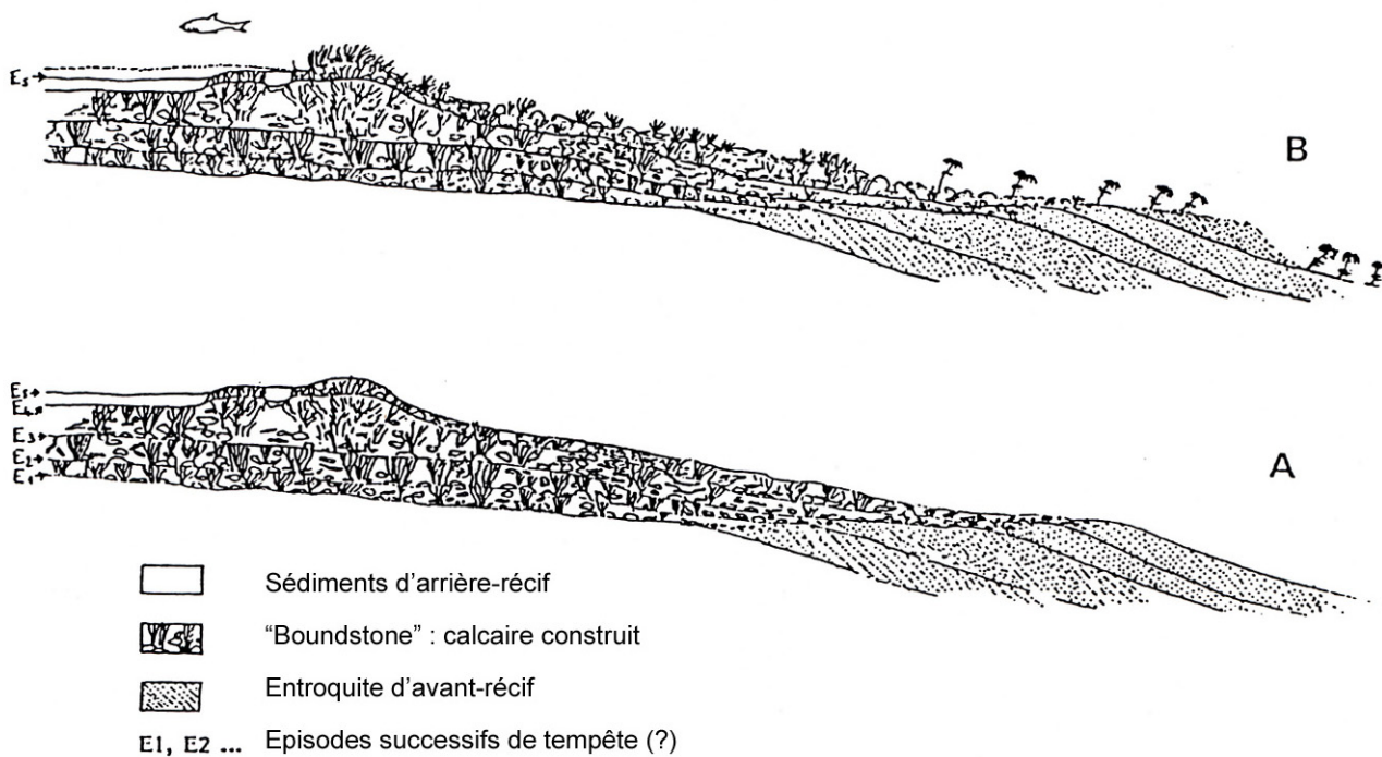
Modèle de sédimentation des formations récifales de l'Oxfordien moyen à Haudainville
