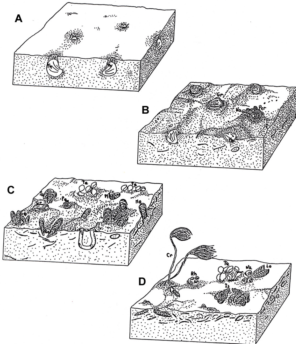
Reconstitution du changement de faune lors de l'évolution d'un fond mou (A) en fond durci (D) - sommet du Terrain à Chailles. D'après Poirot (1987)
