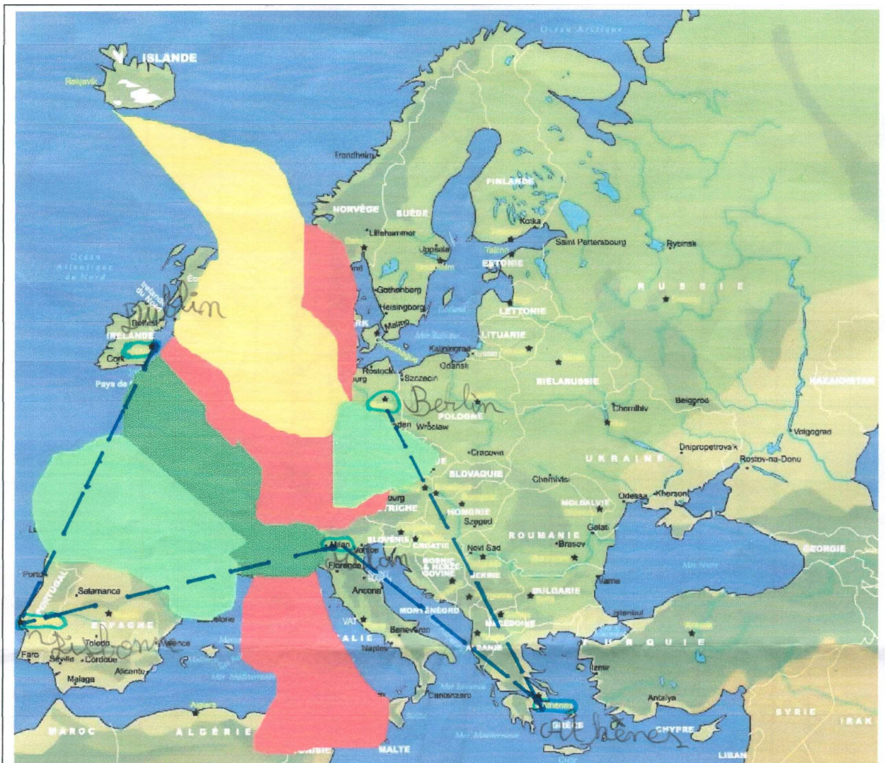
ZONES DE POUSSIÈRES VOLCANIQUES SUR L'EUROPE
