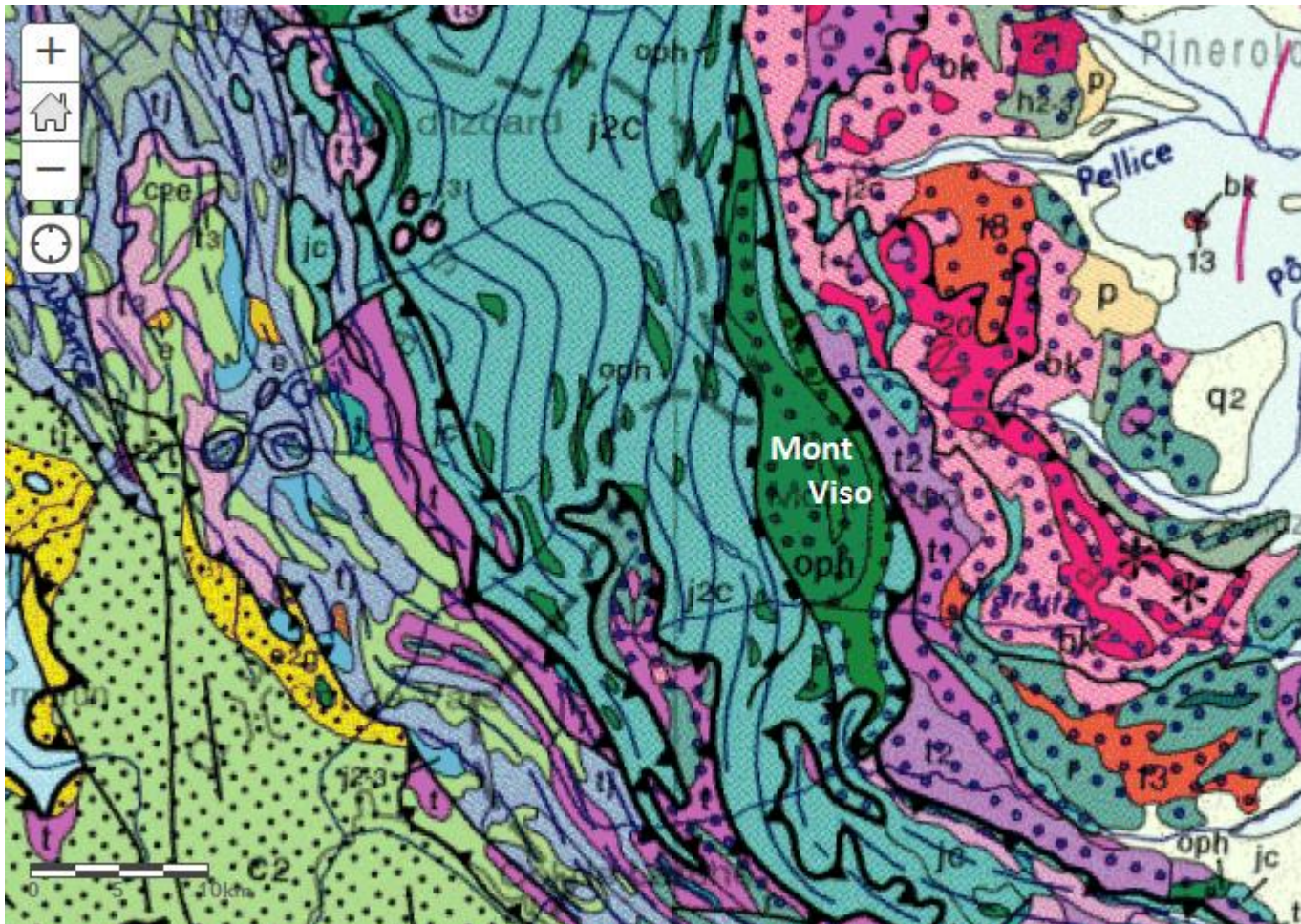
Extrait de la carte géologique de la France au millionième et localisation du secteur du Mont Viso (BRGM, Esri)
